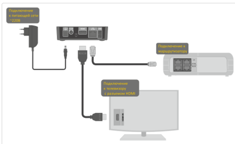
Рисунок 11 – Пример подключения медиацентра NV-100/NV-102
